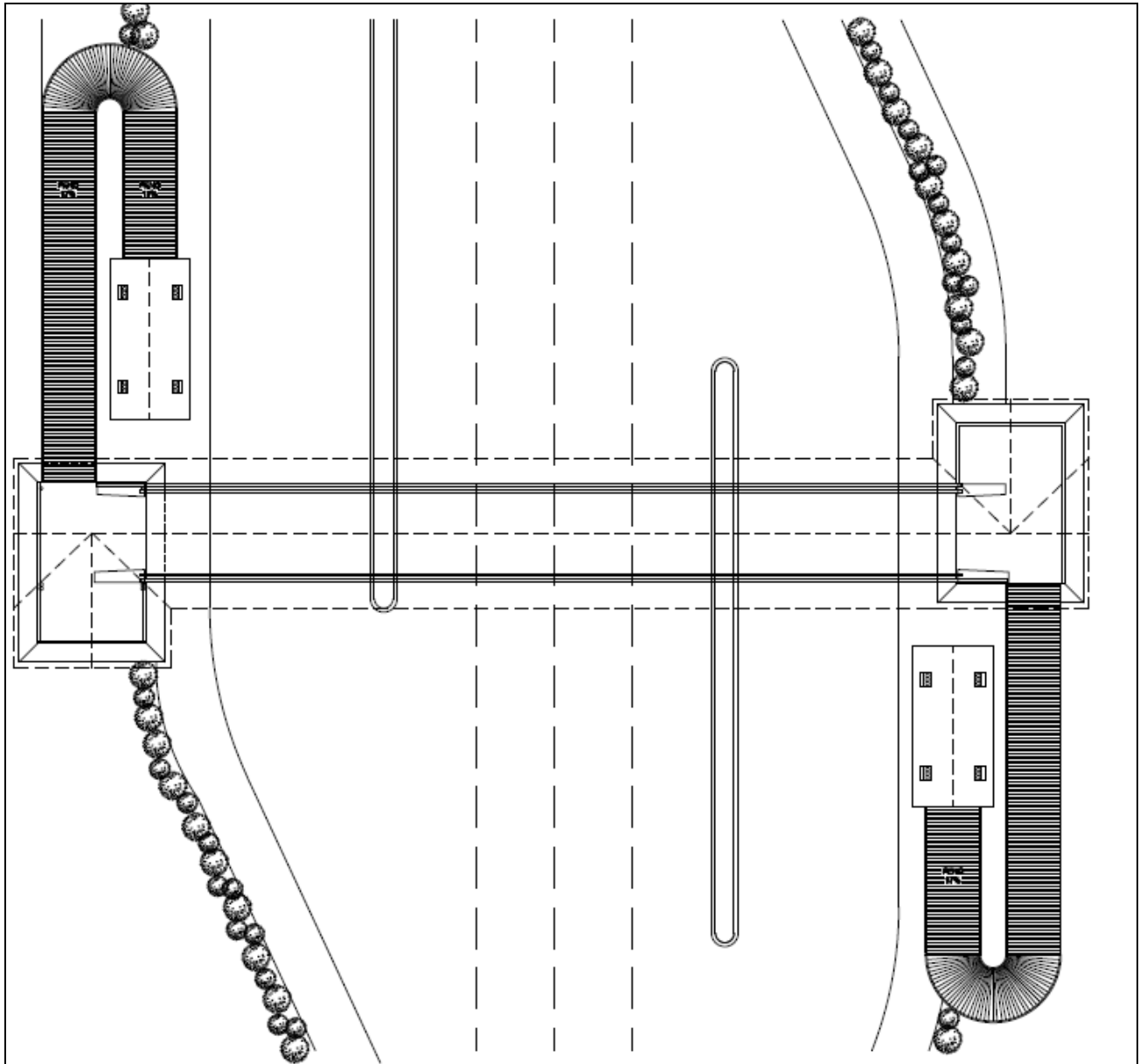
Planta general del puente sobre la vía al Lago de Atitlán. se accede de los dos lados de la finca por medio de rampas peatonales
